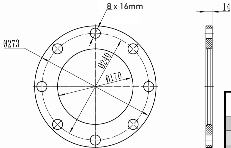
Dimensiones Brida con 8 Bárenos de 16mm
