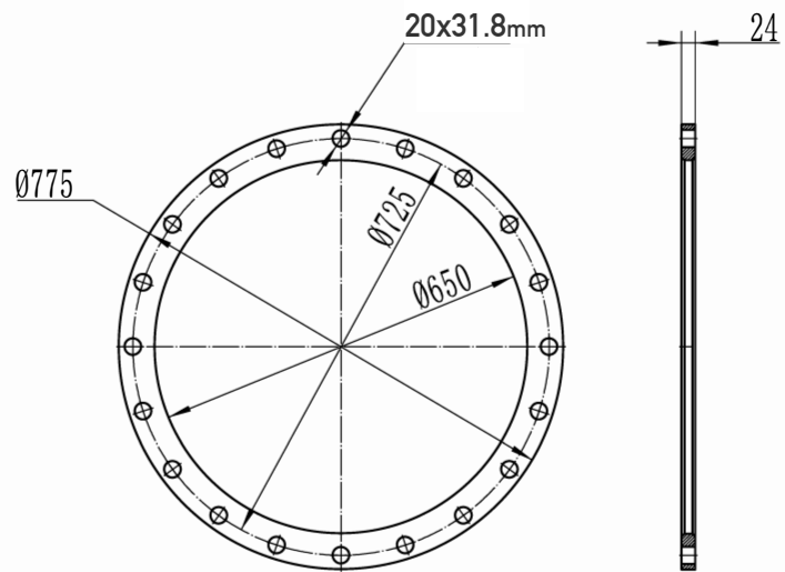
Dimensiones Brida con 20 Bárenos de 31.8mm
