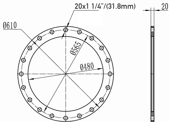
Dimensiones Brida con 20 Bárenos de 1 1/4" / 31.8mm
