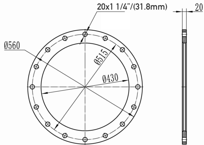
Dimensiones Brida con 20 Bárenos de 1 1/4" (31.8mm)
