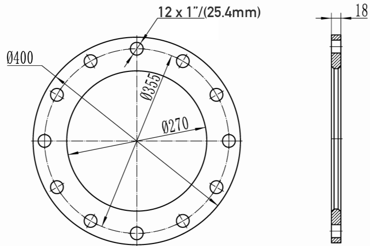
Dimensiones Brida con 12 Bárenos de 1" / (25.4mm)
