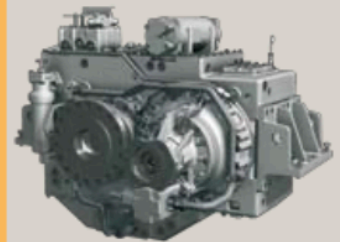
ZF 9000 NR2HL
